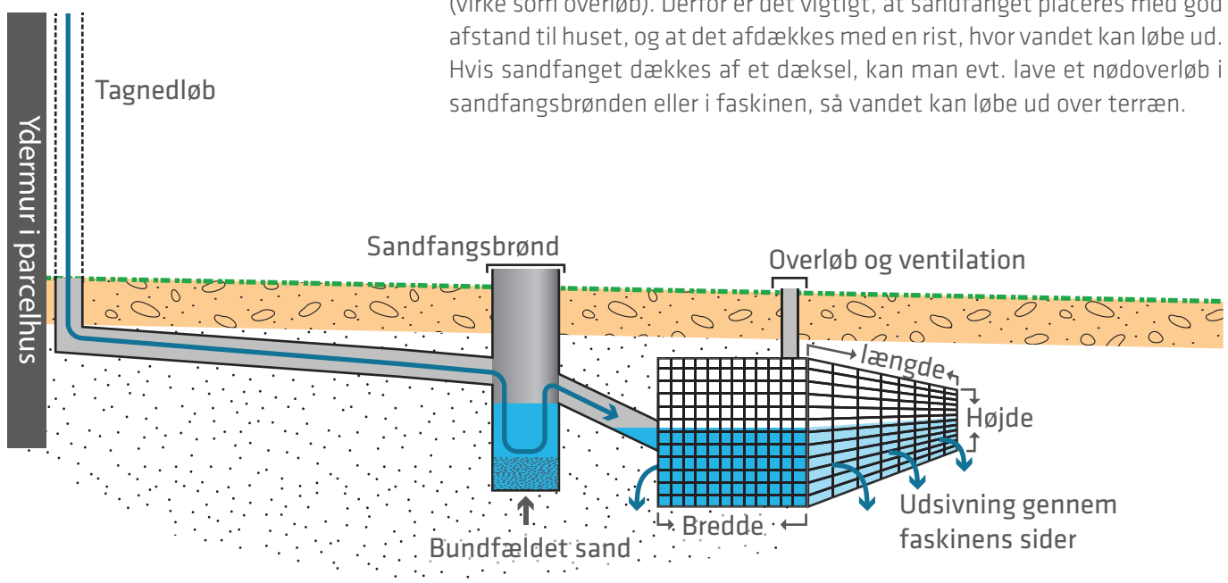
Figur 16: Principssnit for afledning af regnvand til nedsvivning i faskine. Regnvandet ledes fra nedløbsrøret via sandfangsbrønden til faskinen. Illustration Orbicon
